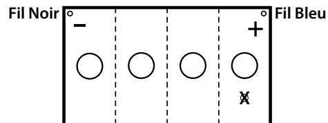
Exemple d'une installation sur un ensemble de batteries 8V. ✕ indique la zone de perçage.
