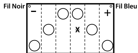
Exemple d'une installation sur un ensemble de batteries 12V. ✕ indique la zone de perçage.
