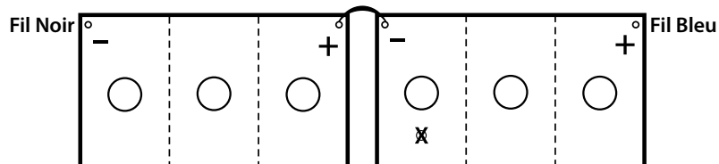
Exemple d'une installation sur deux batteries 6V. ✕ indique la zone de perçage.
